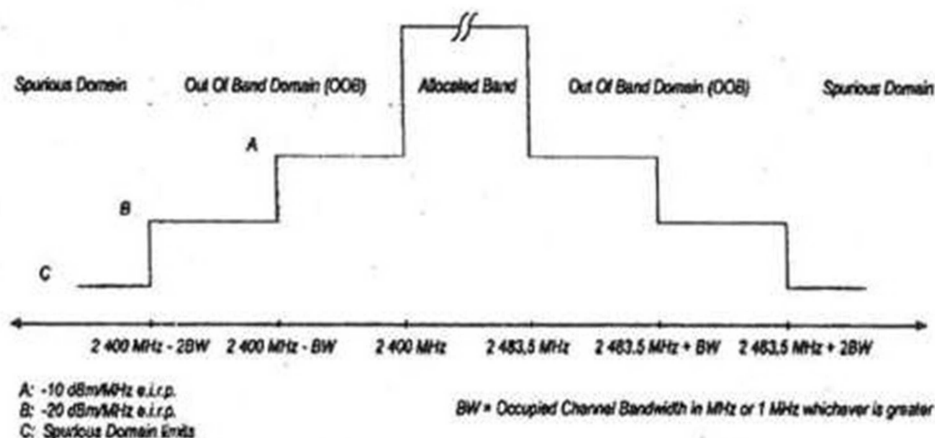
Gambar 1. Transmit Mask (ETSI 300. 328)
