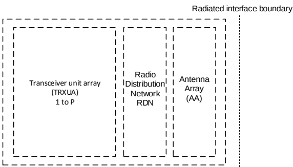
Gambar 1. Titik referensi ( reference points ) untuk pengukuran radiated pada BS type 2-O.
