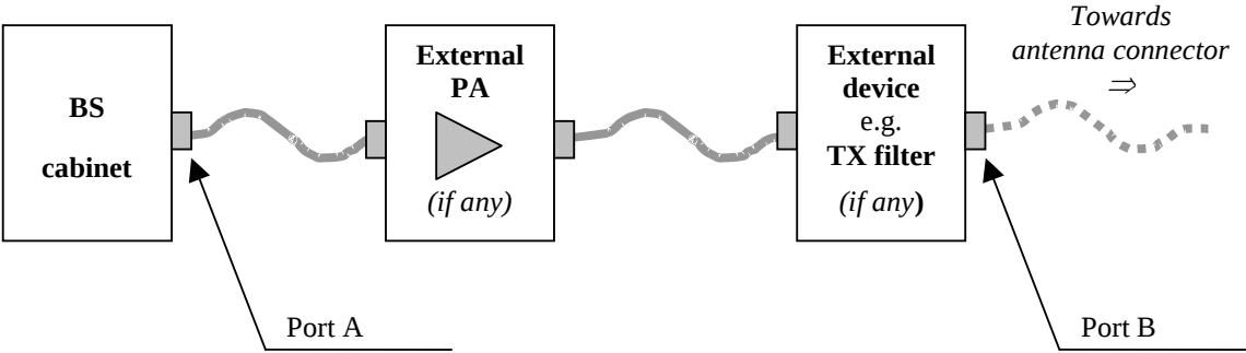
Gambar 1. Interface pemancar BS type 1-C.
